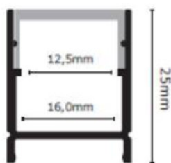
Leuchtenprofil
